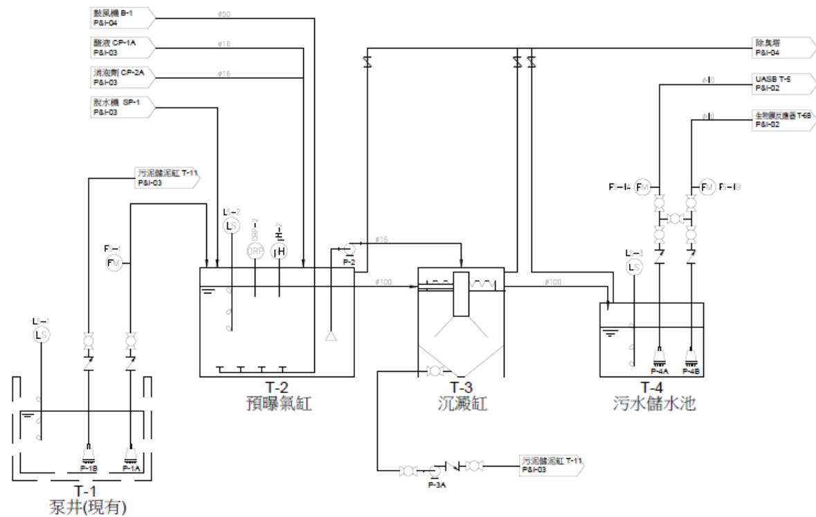
先進預處理系統
