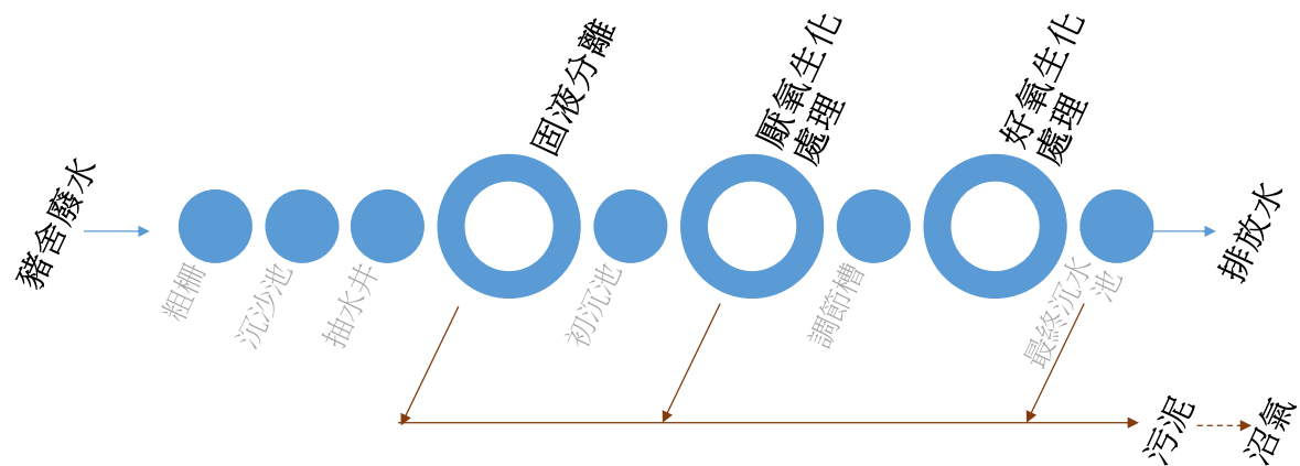
圖表 1.2 傳統三段式豬糞尿廢水處理系統
