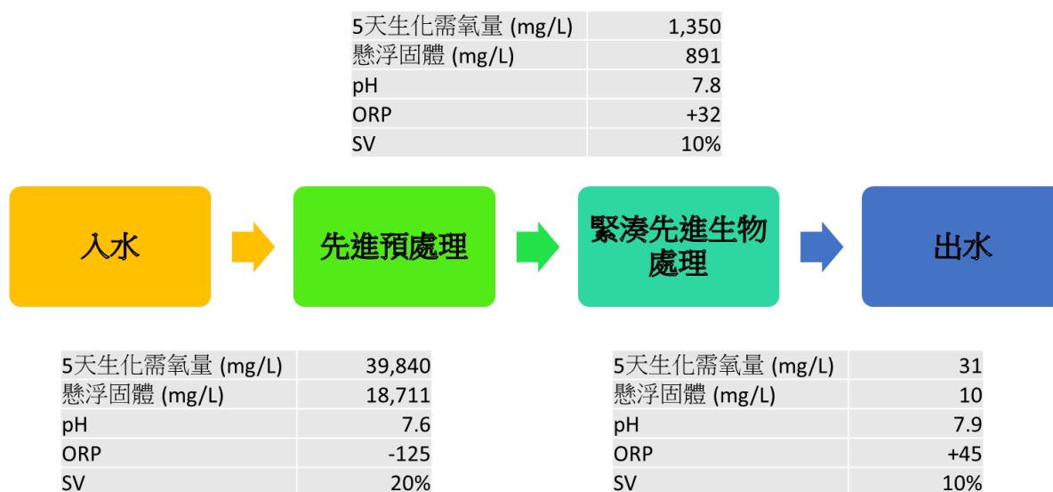
圖表 7.2 獨立單元的水質和運行參數
