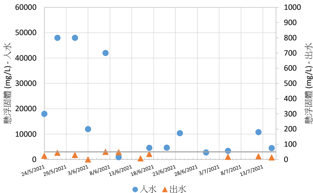
圖表 7.6 2021/05/24 至 2021/07/15 期間懸浮固體變化
